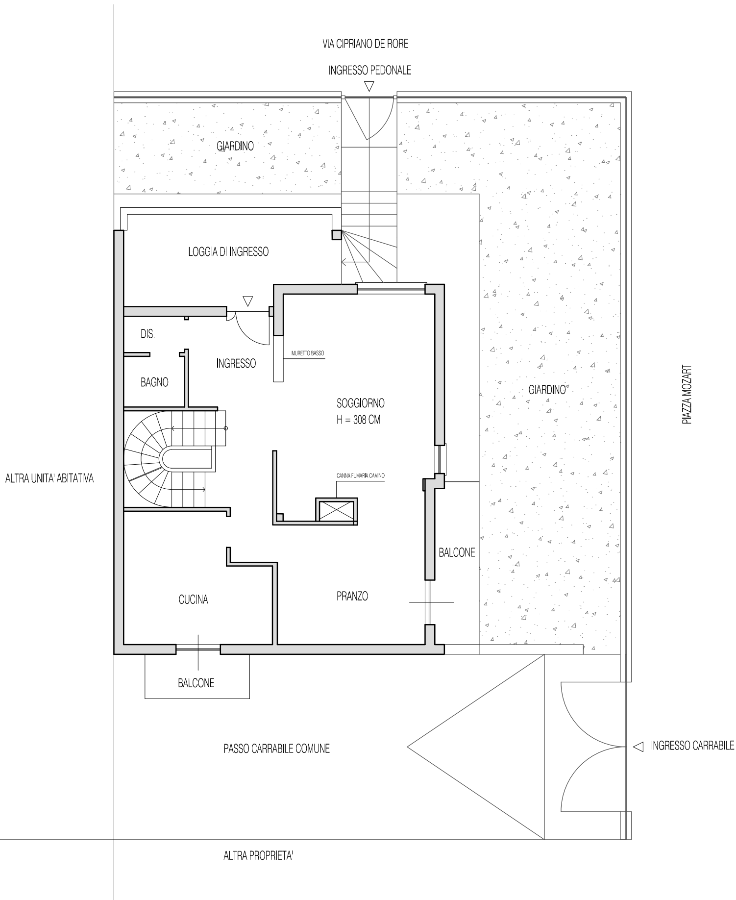
PIANTA PIANO TERRA H = 308 CM
